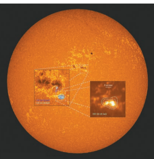
圖為「夸父一號」太陽硬X射線成像儀（HXI）在2022年11月11日觀測到的一個C級耀斑硬X射線成像與AIA/SDO紫外1700圖像的比較。 中新社
